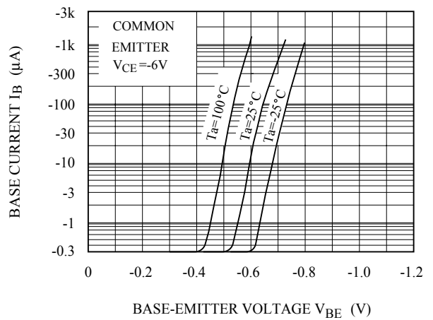
I_B - V_{BE}
